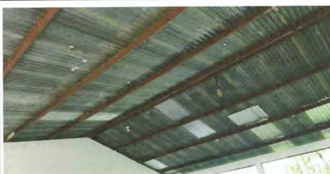
Foto 2: Se observa el desgaste de de la estructura metalica de las aulas del módulo 3 y 1 aula del módulo 4.
